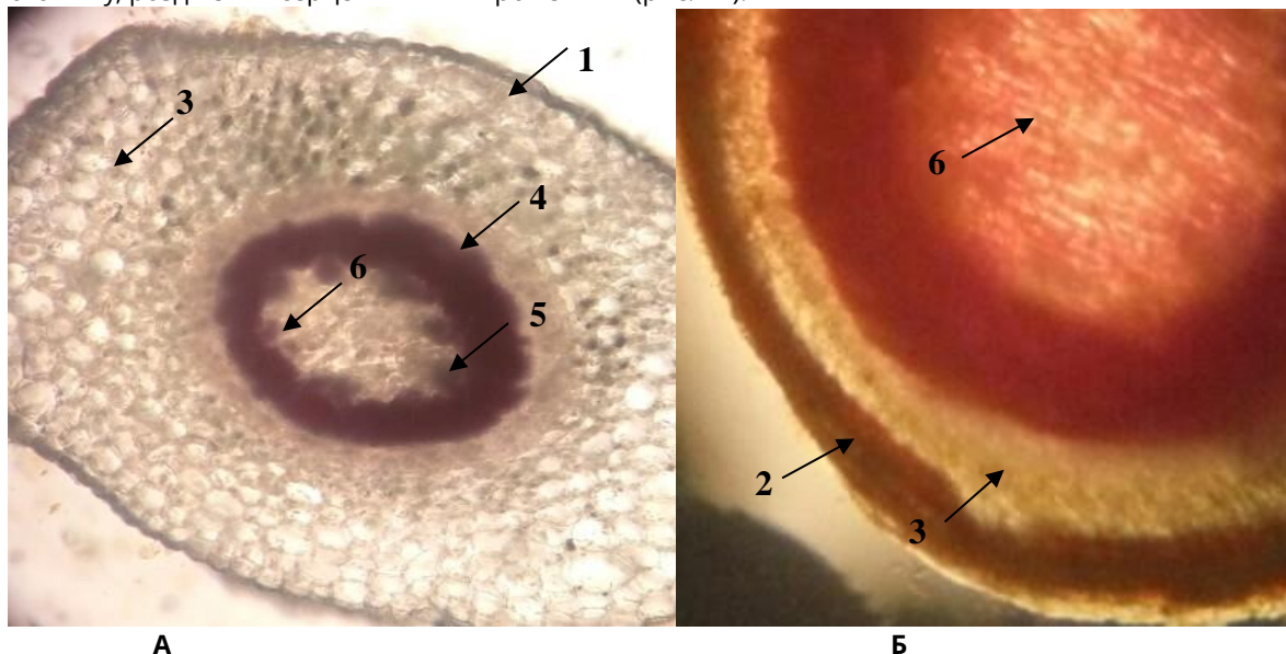
Рис. 1. Поперечний переріз стебла C. socialis (А) та C. perforata (нижня частина) (Б) (збільшення 10 x 4): 1 – епідерма, 2 – коленхіма, 3 – паренхіма первинної кори, 4 – перицикл, 5 – суцільне кільце судинно-волокнистих пучків, 6 – серцевина
