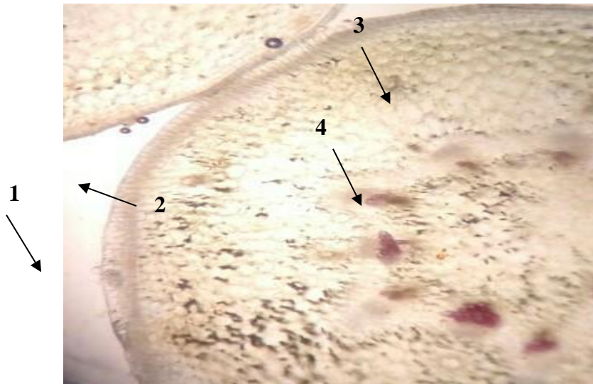
Рис. 5. Поперечний зріз стебла S. rowleyanus (збільшення 10 x 4): 1 – епідерма, 2 – колєнхіма, 3 – корова парєнхіма, 4 – центральний циліндр
